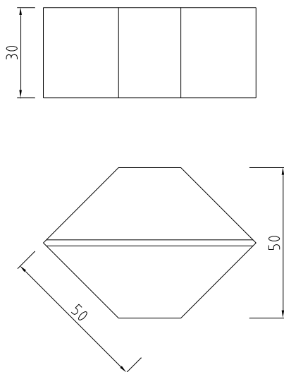
Figura 1 – Configuração da cabeça de manobra
